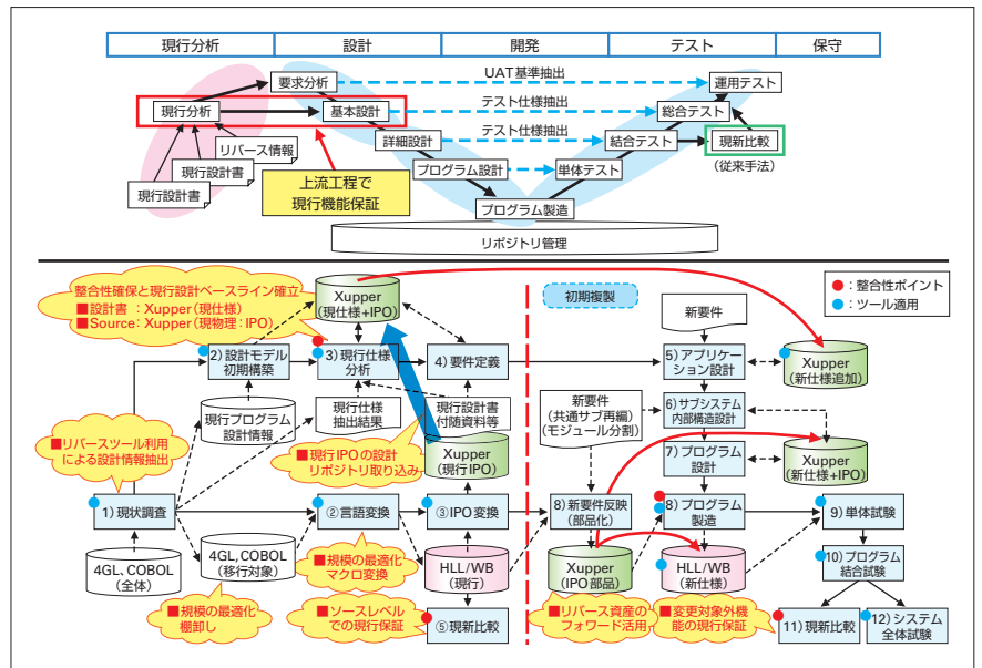
図1：Nモデル 開発工程実装イメージ（Nモデルによる現行保証と最適化開発方式）
